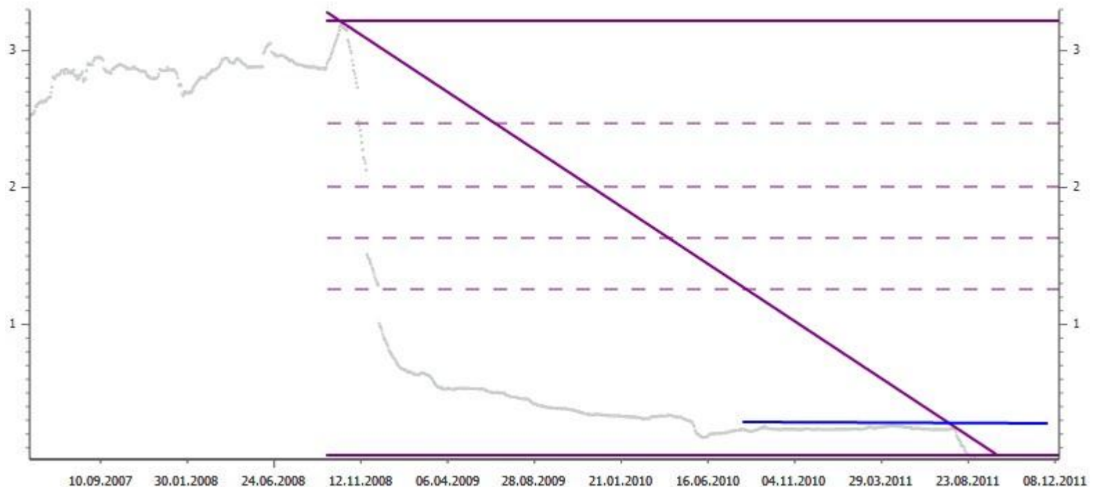
LIBOR CHF - LIBOR 6 Mts./CHF: 15.05.2007 - 13.12.2011
